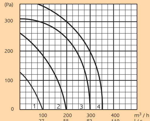
Puhaltimien vapaapuhalluskäyrät
