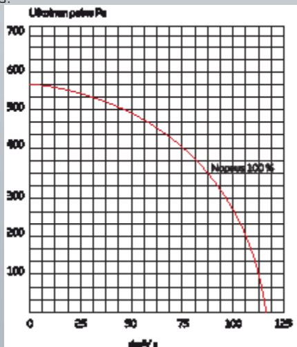
Puhallinkäyrä
