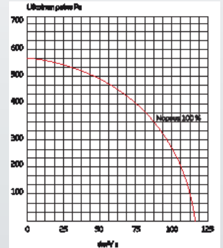
Nilan VPL15C
