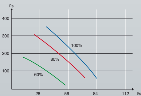
Tuloilmavirta
