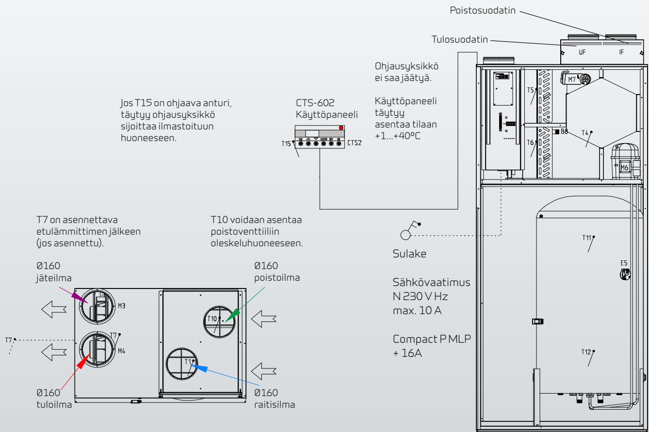
Kuva 2: Anturien sijainti Compact P -laitteissa
