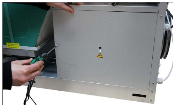
4. Laitteen etuosan sähkötilan suojapelti irroitetaan.
