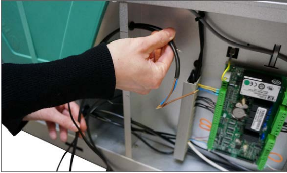
7. Termostaatin B3 ja T9 anturin johdot vedetään läpiviennin läpi kytkentätilaan. Kytkeä pääpiirikortille ja muuntajaan kytkentäkaavion mukaisesti. Kiinnitä suojapelti takaisin paikalleen, muista maadoitusjohto.
