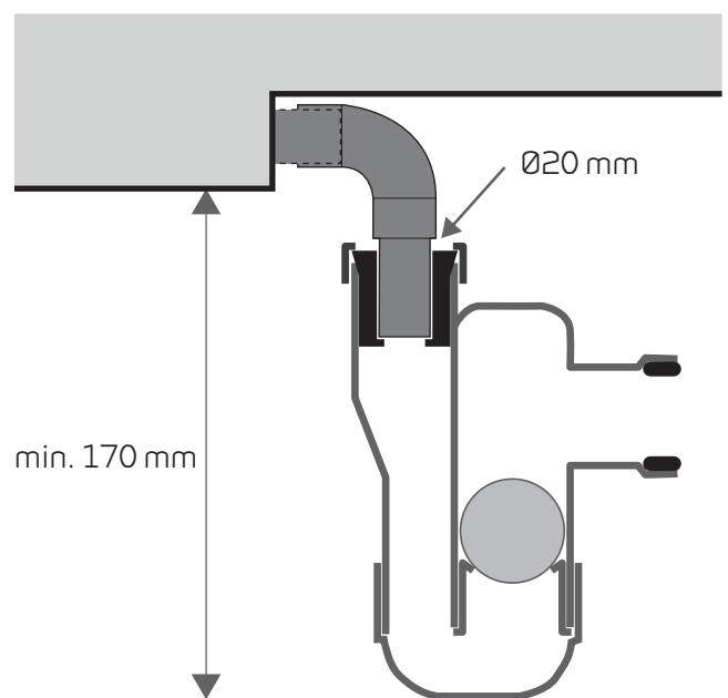
Nilan pallovesilukon kytkentä
