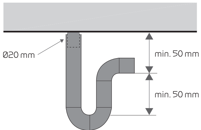
Vesilukon kytkentä yleensä
