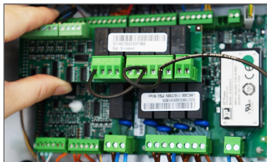
4. Paina laajennuskortti oikeaan kohtaan pääpiirikortilla.
